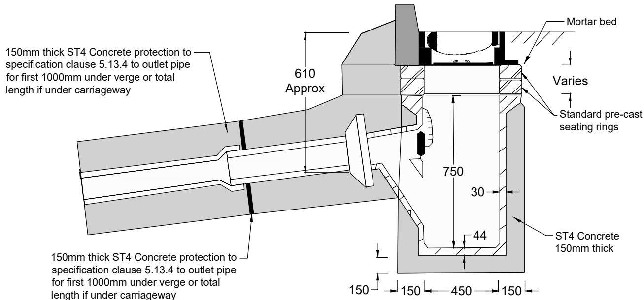
TYPE G5 TRAPPED ROAD GULLY N.T.S.
